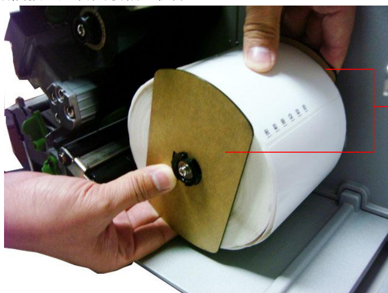
紙卷軸擋板
